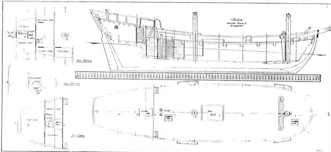
DECK DETAIL CHALEUR
