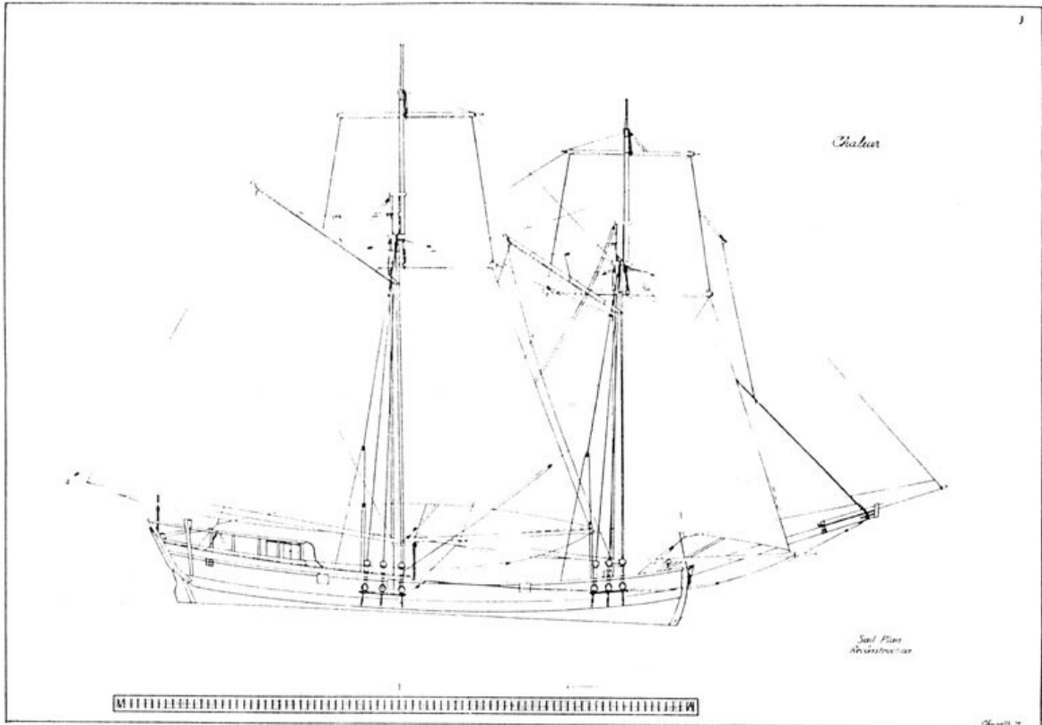
SAIL PLAN CHALEUR
